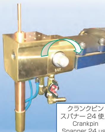
前面アタッチメント部 Front attachment part
